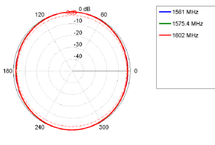
XY Plane: 1561-1602 MHz
