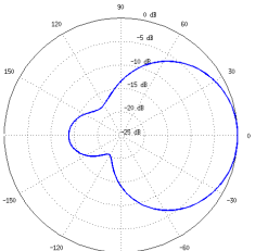
V-Pol Elevation
